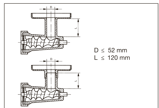
Bild 4: Wolf mit fester bzw. abnehmbarer Schüssel. Erforderliche Sicherheitsabstände.
