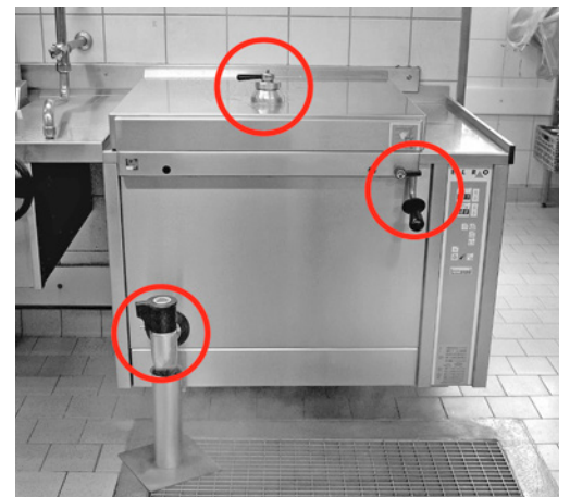
Bild 5: Sicherheitselemente am Kessel.
